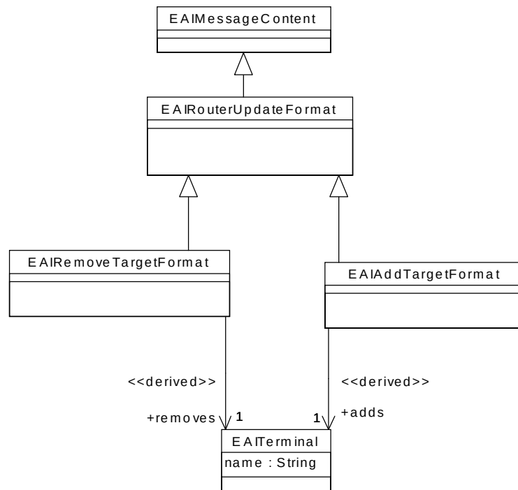
Figure 6-34 EAIRouterUpdateFormat
