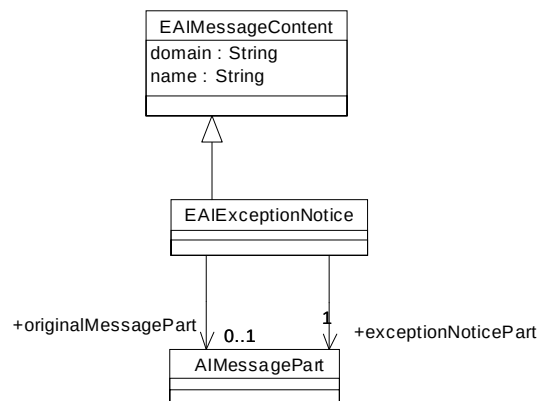
Figure 6-11 EAExceptionNotice
